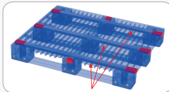
Längsverstärkung
